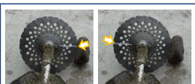
a. チップソー横に石を1mm離して置き、 刃を半回転させて、その隙間が同じ なら「 芯ブレ無し 」と判断する
