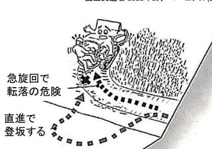
草刈機の走行手順と旋回位置
