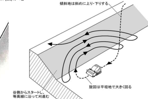
図 1.30 法尻側から平坦地で方向転換して法肩側へ進む
