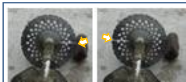
a. 刈刃の横に接触しように石を置き、刃を半回転、手で廻して隙間の量に変化なければ「 芯ブレ無し 」と判断できる
