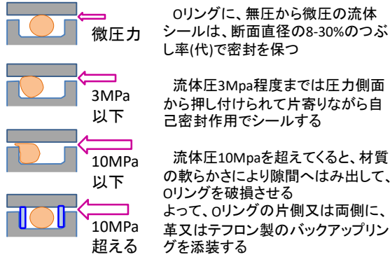
Oリングと溝寸法の設定基準
