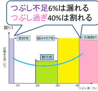
Oリングと溝寸法の設定基準
